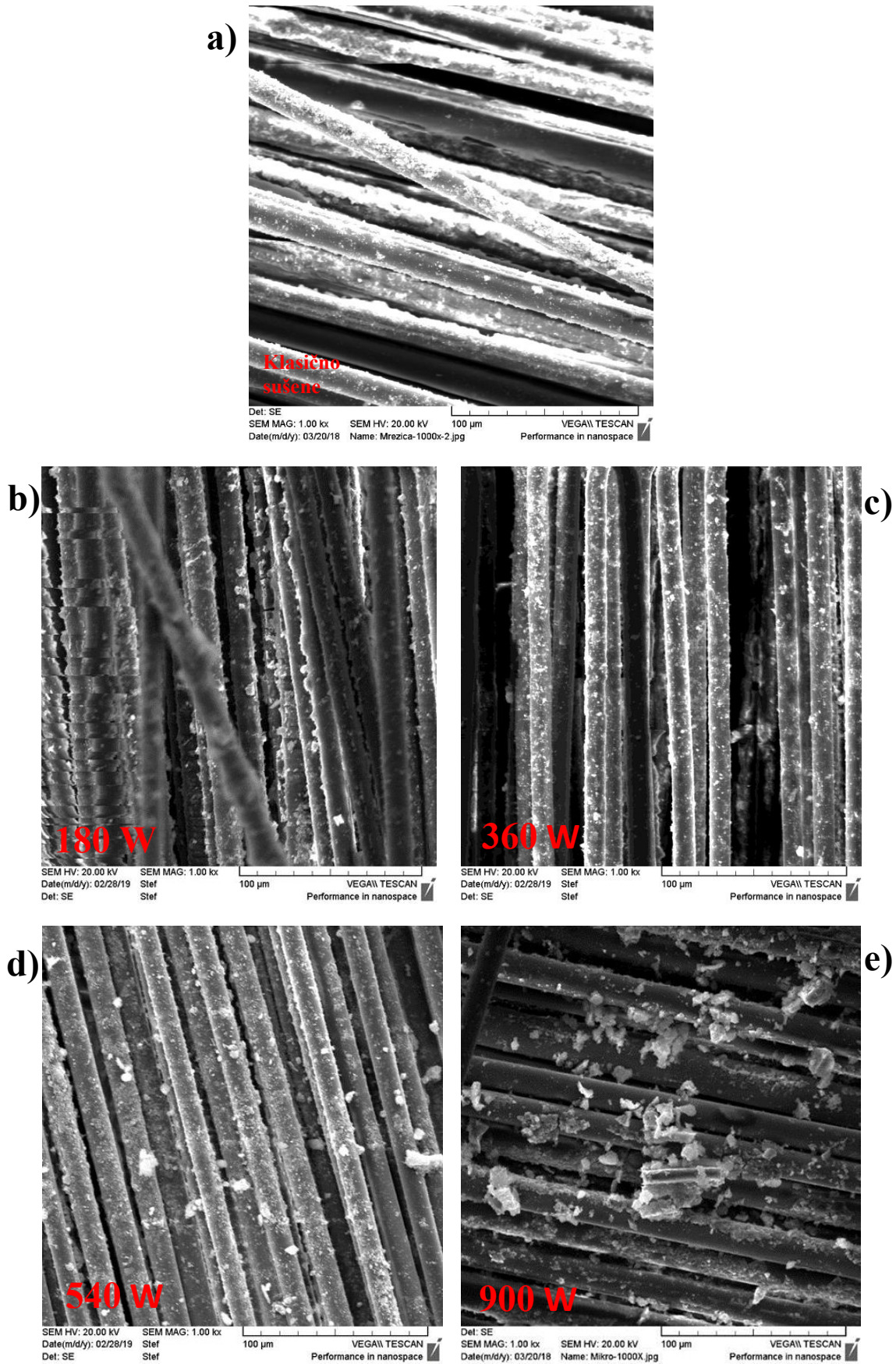
Slika 42 SEM prikaza fotokatalizatora TiO 2 nanosenog na staklena vlakna i sušenog a) klasično te mikrovalno snagom b) 130 W, c) 360 W, d) 540 W i e) 900 W.
