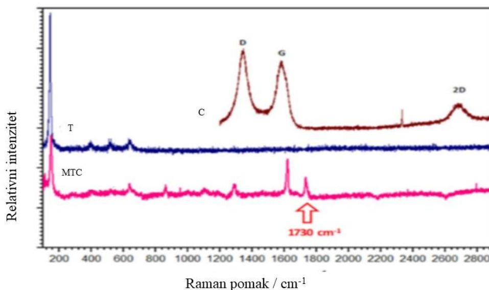
Slika 54 Raman spektri fotokatalitičkih sastojaka i fotokatalitičkih kompozita na staklenoj mrežici [137].
