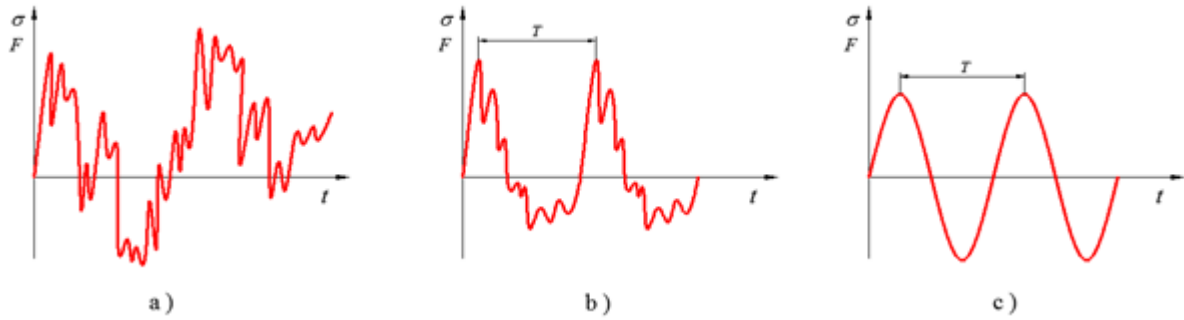
Slika 26 Vrste dinamičkih opterećenja/naprežanja [18]: a) stohastičko, b) periodičko (T-period) i c) harmonijsko
