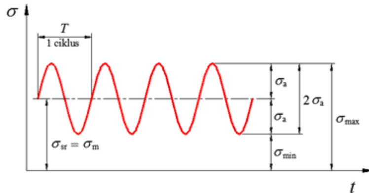
Slika 27 Prikaz harmonijskog naprežanja [18]
