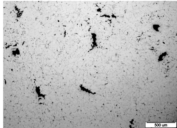
Slika 6. Mikrostruktura kompozita s 4% lebdjećeg pepela u ugnječenom stanju
