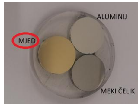
Slika 5. Izrezani i zaliveni uzorci
