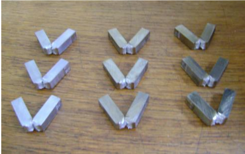
Slika 6. Ispitni uzorci nakon ispitivanja na Charpyjevom batuu
