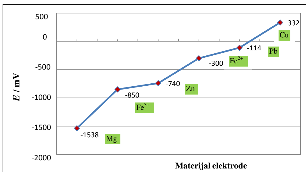
Slika 3. Elektrokemijski niz („Voltin niz“) ispitanih metala u odnosu na \text{Ag} | \text{Ag}^+ elektrodu
