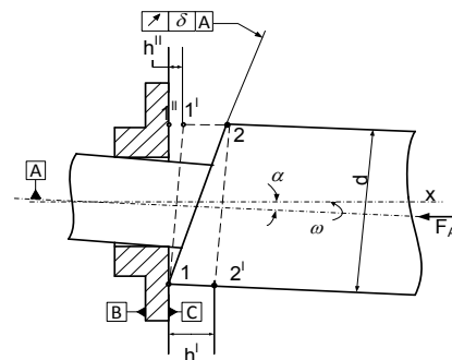
Фиг. 2 Схема на вала и опорната шайба
