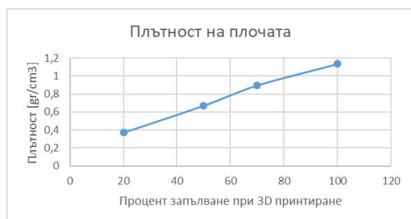
Фиг.2 Плътност на плочата при различен коефициент на запълване при 3д принтирането и.
