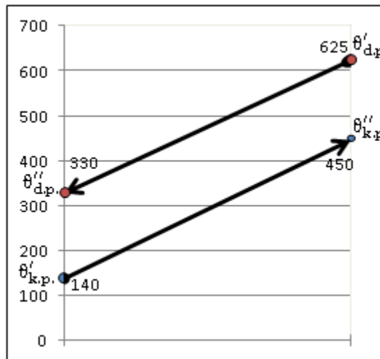
Slika 28. Prikaz promjene temperatura u drugoj sekciji
