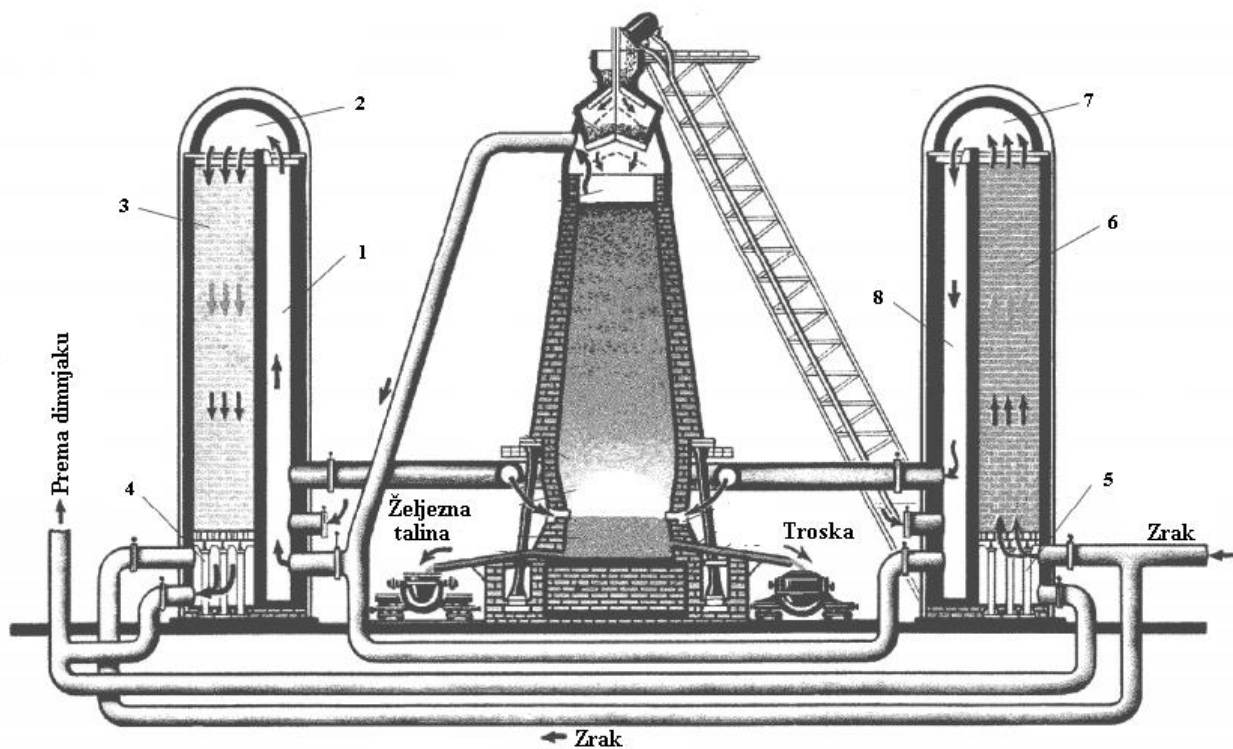
Slika 6. Shematski prikaz kaupera za zagrijavanje zraka [18]
