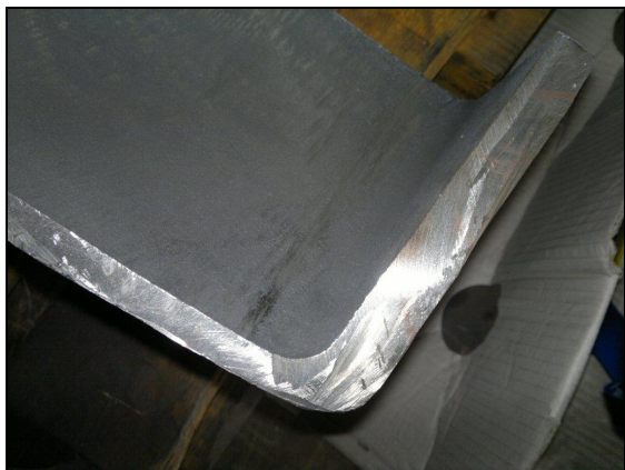
Slika 4.2. Kućište filtra KSF DN200 presječeno po visini radi ispitivanja poroznosti
