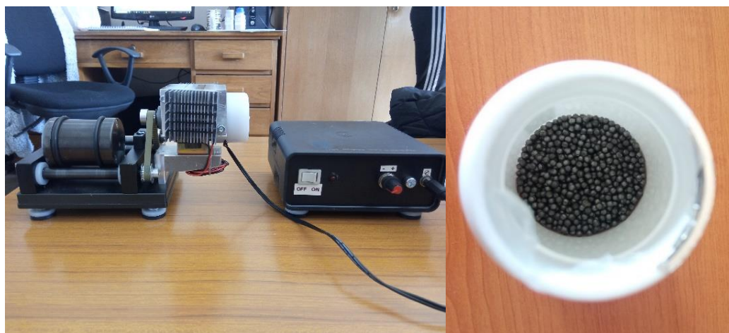
Slika 15. Kuglični mlin i kuglice za miješanje
