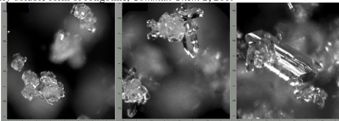
Slika 1. Polimorfni prijelaz API-ja forme A u formu B snimljen procesnim mikroskopom Blaze 900
