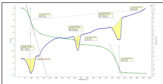
Fig. 11 DTA - MAPEI Indrocrete KR1000
