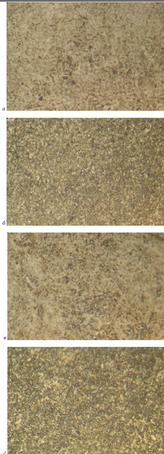
а - ковка, закалка 880 °С + отпуск 200 °С; б - ковка, закалка 880 °С + отпуск 500 °С; в - отжиг, закалка 880 °С + отпуск 200 °С; г - отжиг, закалка 880 °С + отпуск 500 °С
