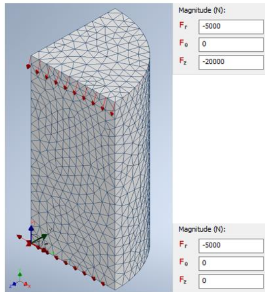
Slika 41. Definiranje opterećenja
