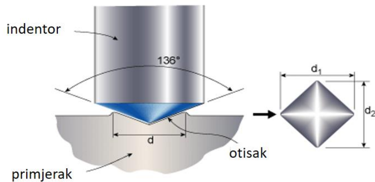
Slika 12. Utiskivanje indentora [22]
