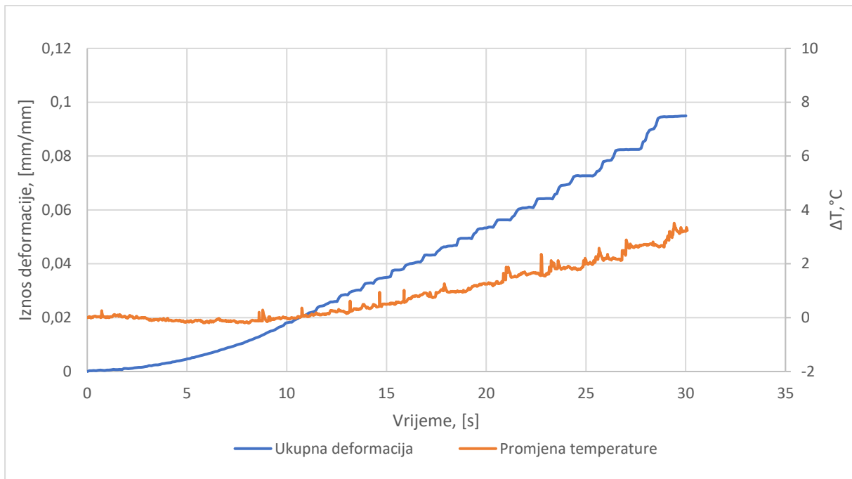
Slika 46. Usporedni dijagram temperaturene promjene i DIC analize deformacije primjer 2
