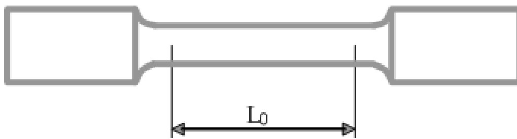
Slika 17. Prikaz uzorka za statičko vlačno ispitivanje, L_0 označava mjerni dio ispitnog uzorka [51]
