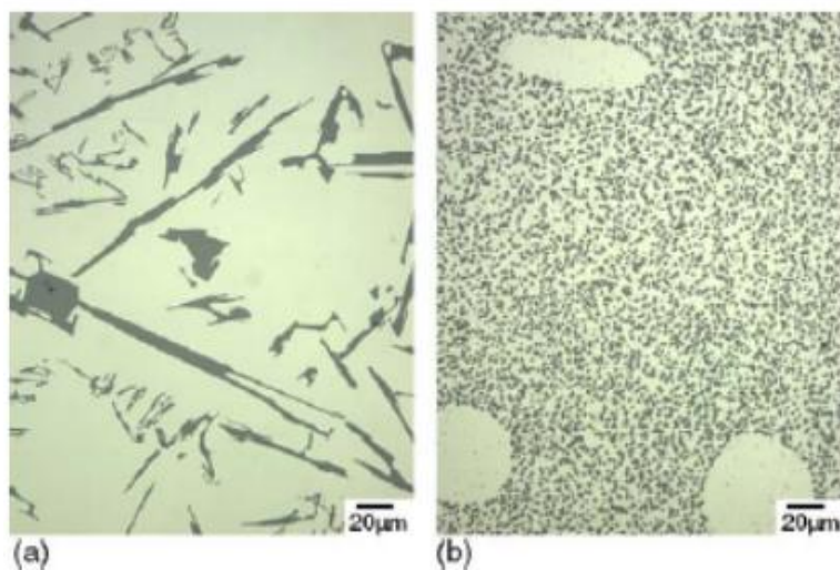
Slika 35. Usporedba morfologija eutektičke Si faze [22] a) nemodifikirana lamelarna struktura b) struktura modifikirana dodatkom Sr = 300 ppm
