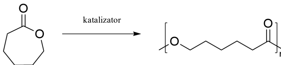
Slika 14. Sinteza polikaprolaktona [38]
