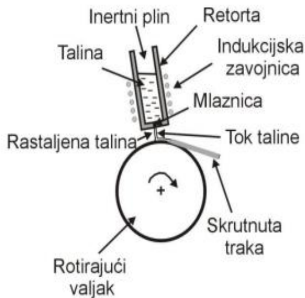
Slika 6. Shematski prikaz „melt spinning“ metode
