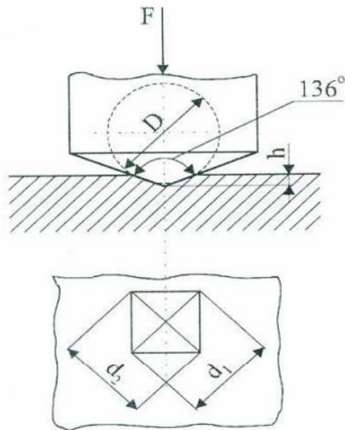
Slika 5.16. Shematski prikaz mjerenja tvrdoće [11]
