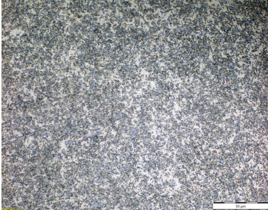
Slika 6.8. Mikrostruktura uzorka 3, 1390 °C
