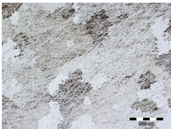
Slika 54. Optičke mikrofotografije ruba uzorka 3 (0,75 % Zr) nakon toplinske obrade ( 900\text{ }^{\circ}\text{C}/15\text{ min/voda} ); a) 50x, b) 100x, c) 200x, d) 500x
