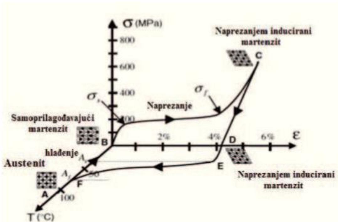
Slika 16. Dijagram naprezanje-deformacija-temperatura Nitinol legure s prijetljivosti oblika [14]
