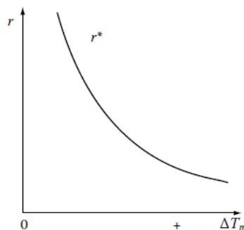
Slika 9. Promjena kritičnog radijusa nastajanja nukleusa s pothlađenjem [16]
