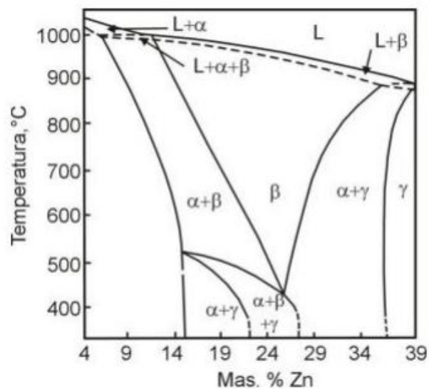
Slika 4. Ravnotežni fazni dijagram ternarne legure CuZnAl s vertikalnim presjekom pri 6 % mas. Al [7]
