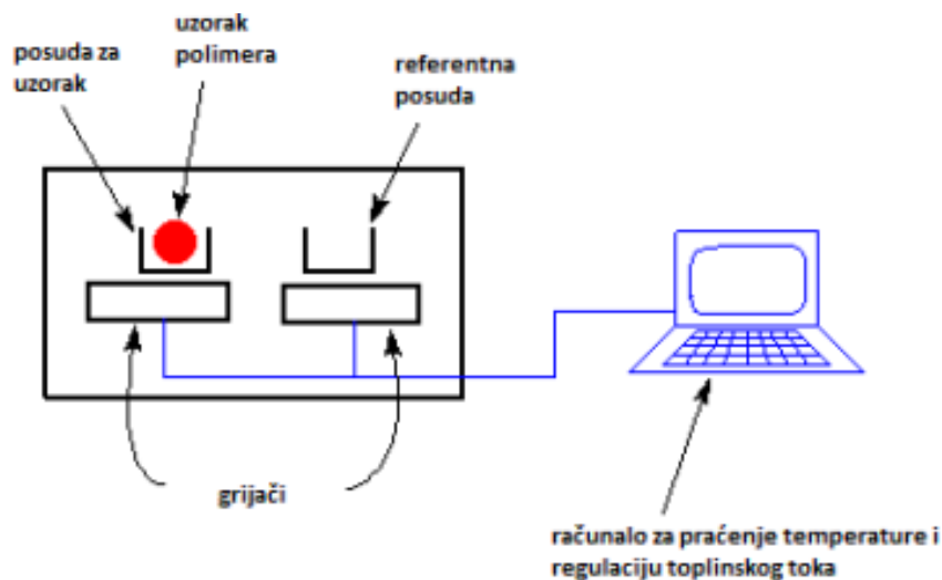
Slika 15. Shema DSC instrumenta [30]
