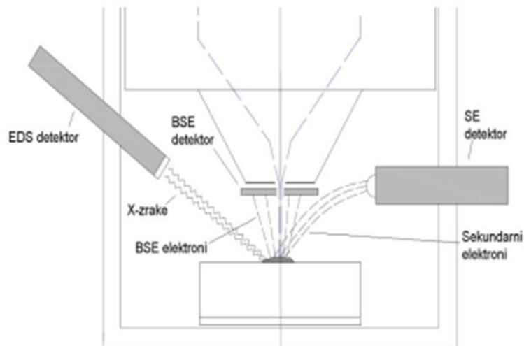
Slika 17. Shematski prikaz osnovnih vrsta detektora [34]
