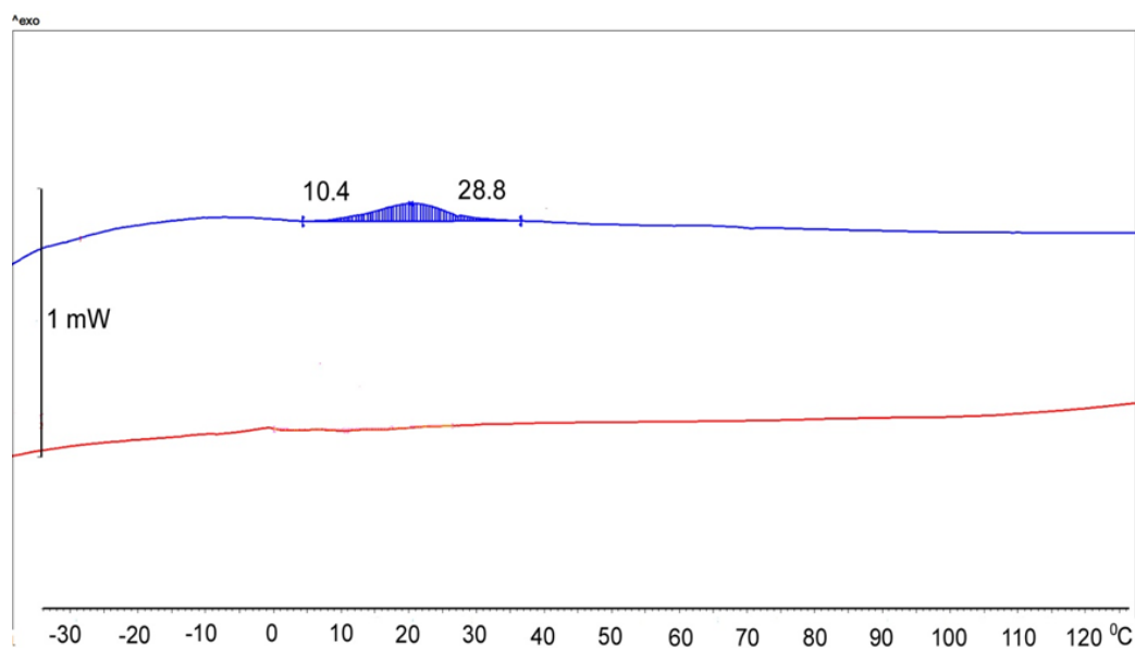
Slika 42. DSC termogram za Cu-Al-Mn leguru pripremljenu u indukcijskoj peći
