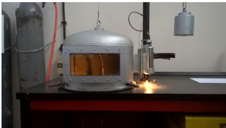
Slika 19. Elektrolučna peć
