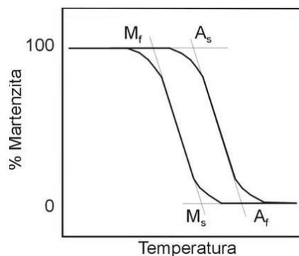
Slika 10. Histereza u SMA legurama [6]
