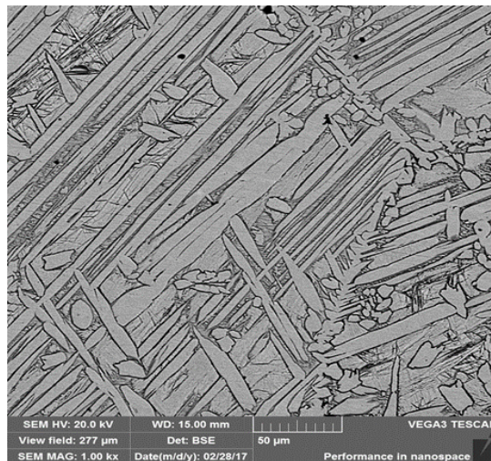
Slika 35. Mikrofotografije CuAlMn legure u lijevanom stanju nakon pripreme u: a) elektrolučnoj peći, b) indukcijskoj peći (povećanje 1000x)
