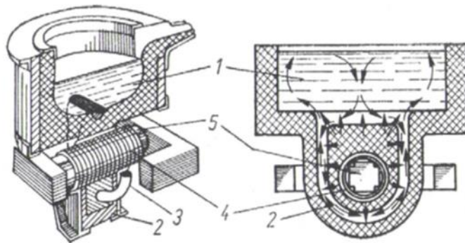
Slika 13. Shematski prikaz indukcijske peći: 1-metal, 2-obloga, 3-kanal, 4-svitak, 5- jezgra [28]
