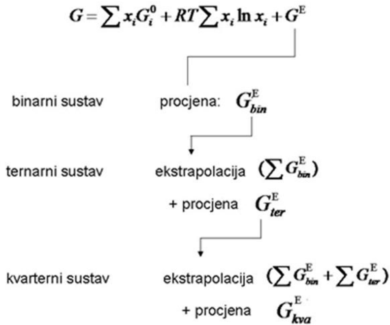
Slika 18. CALPHAD metodologija [36]
