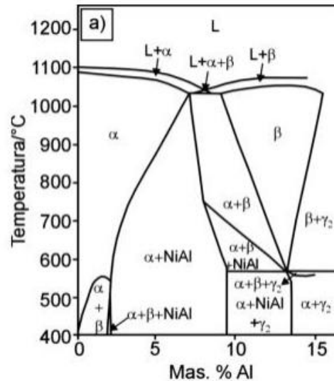
Slika 5. Ravnotežni fazni dijagram za leguru CuAlNi pri vertikalnom presjeku od 3 mas.% Ni [5]
