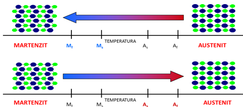
Slika 9. Transformacije SMA legura [21]
