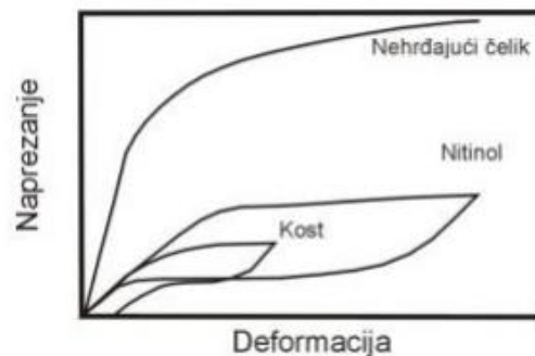
Slika 1. Shematski prikaz krivulje naprezanje – deformacija [6]
