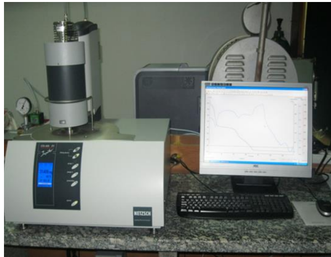
Slika 30. Uređaj za simultanu toplinsku analizu, STA DSC/TG NETZSCH
