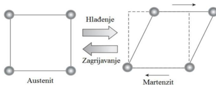
Slika 7. Promjena oblika jedinične ćelije tijekom martenzitne transformacije [19]
