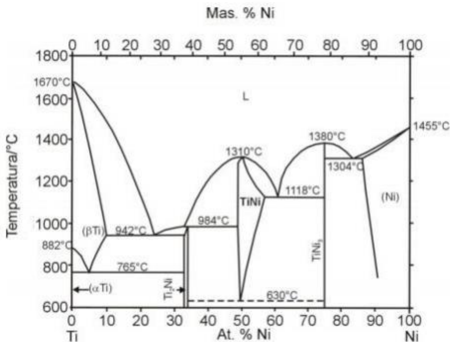
Slika 2. Fazni dijagram NiTi legure [7]
