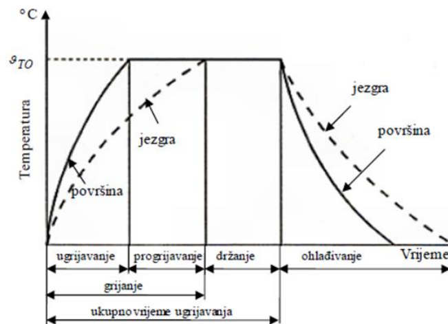
Slika 14. Dijagram ovisnosti promjene temperature o vremenu [29]
