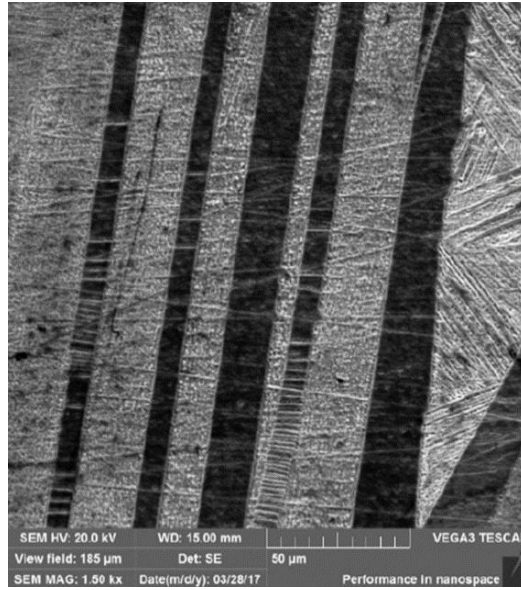
Slika 40. SEM mikrofotografije mikrostrukture nakon kaljenja za: a) Cu-10Al-8Mn leguru, b) Cu-10Al-8Mn-4Ag
