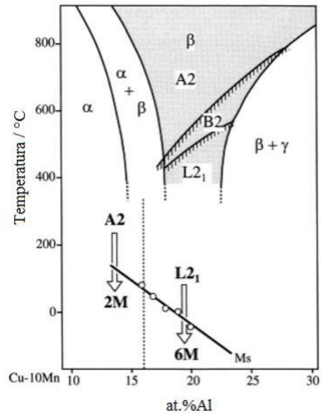
Slika 6. Vertikalni presjek Cu-Al-Mn legura pri 10 at.% Mn [16]
