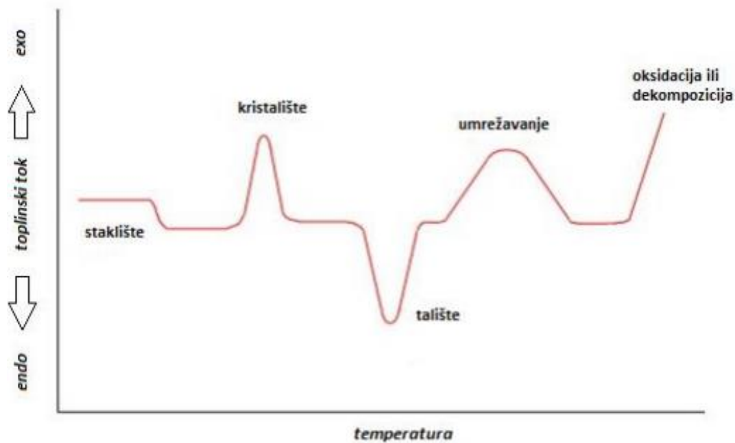
Slika 16. DSC termogram [30]
