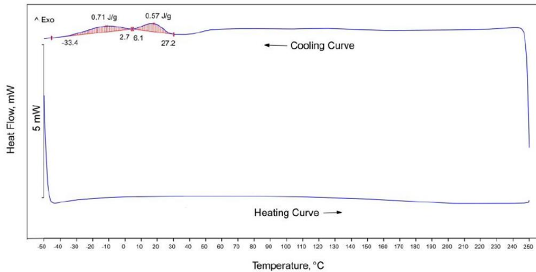
Slika 43. DSC krivulja grijanja i hlađenja za kaljenu leguru Cu-10Al-8Mn-4Ag leguru
