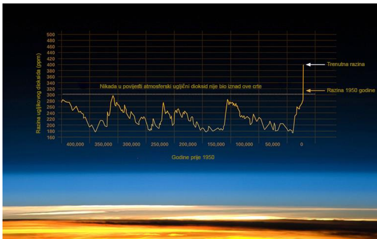
Slika 1. Trend rasta CO 2 [1]
