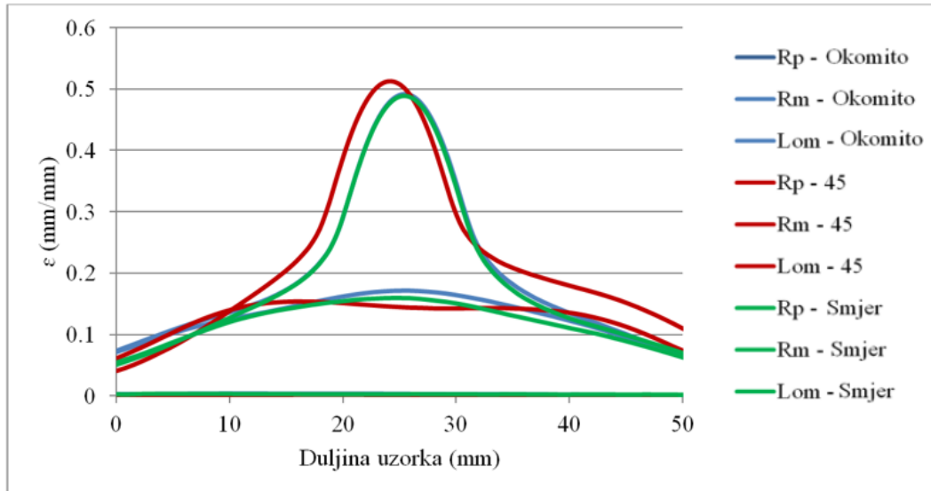
Slika 50. Linijska analiza promjene deformacije u zoni deformacije uzorka toplovaljane trake uzetih u različitim smjerovima u odnosu na smjer valjanja trake
