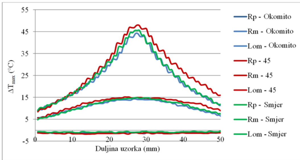
Slika 46. Linijska analiza promjene naprezanja u zoni deformacije uzoraka toplo valjane trake uzetih u različitim smjerovima u odnosu na smjer valjanja trake
