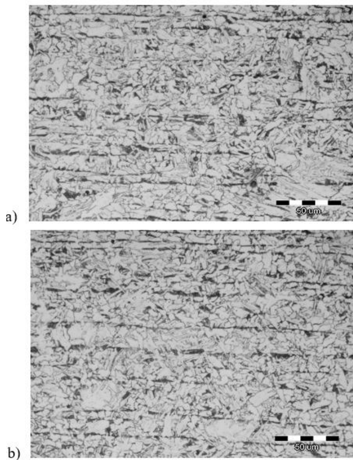
Slika 42. Početna mikrostruktura niskougliječnog čelika u smjeru valjanja ( 0^\circ ): a) okomito na uzorak u smjeru valjanja, b) u smjeru uzorka u smjeru valjanja
