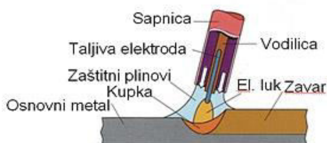
Slika 5. MIG/MAG postupak [7]
