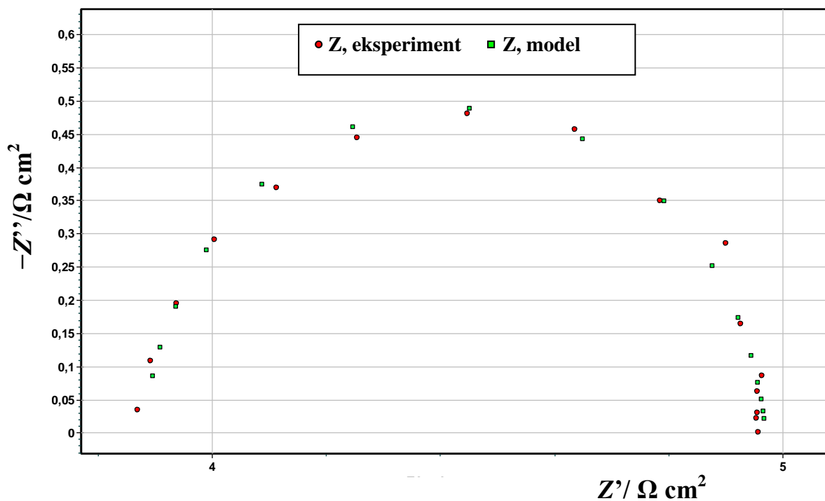
Slika 39. Modeliranje dobivenog Nyquistovog EIS spektra za TRIP-čelik oznake K u mediju 0,5 M \text{H}_2\text{SO}_4 i pri temperaturi od 50^\circ\text{C}
