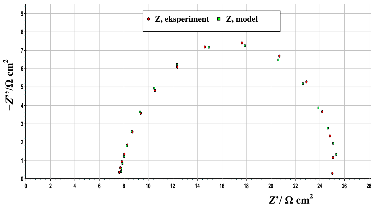
Slika 40. Modeliranje dobivenog Nyquistovog EIS spektra za TRIP-čelik oznake VA u mediju 0,5 M \text{H}_2\text{SO}_4 i pri temperaturi od 20^\circ\text{C}
