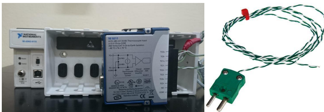
Slika 59. Uređaj za mjerenje temperature
