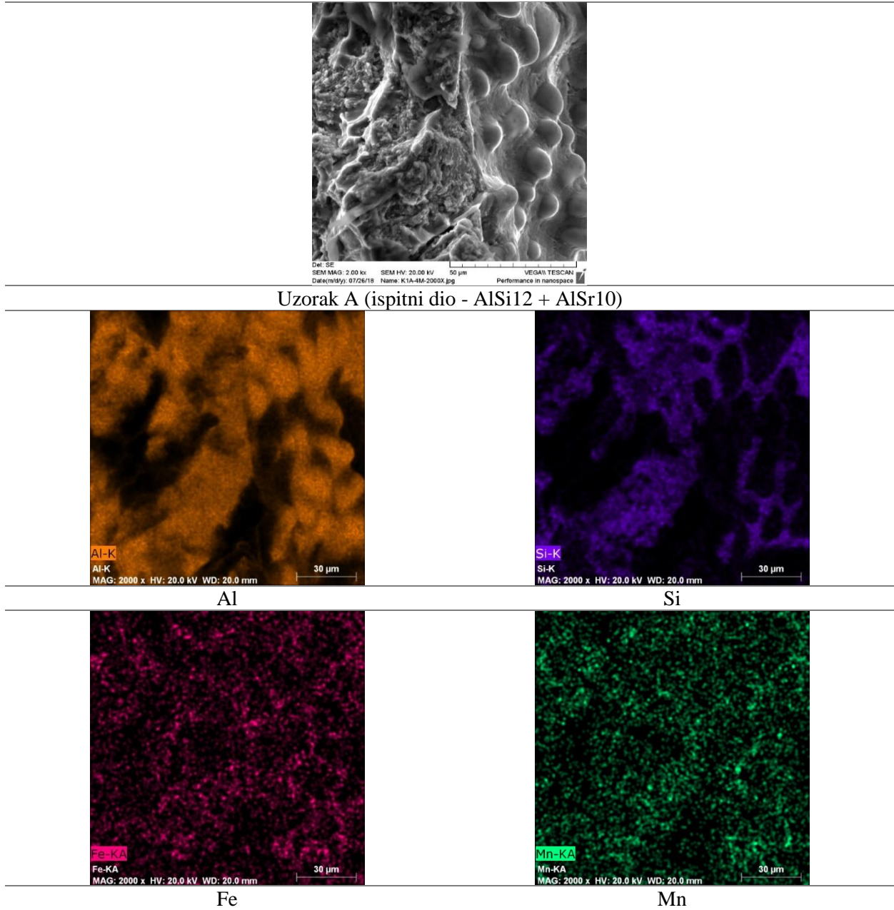
Slika 65. EDS analiza uzorka A
