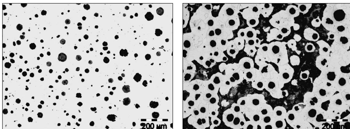
Slika 2.1. Metalografske snimke mikrostrukture feritnog nodularnog lijeva: a) nenagrizenno stanje, b) nagrizenno stanje, nital [7]
