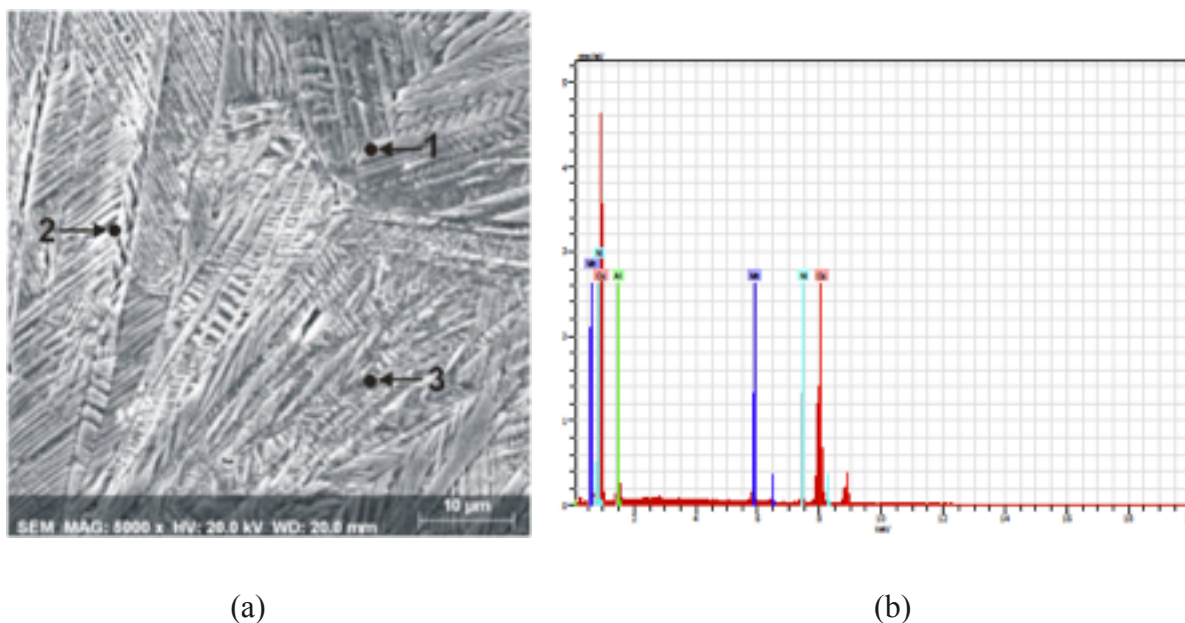
Slika 21. SEM mikrografija (a) i EDS spektar za poziciju 1 (b) Cu-Al-Mn-Ni legure s prisjetljivosti oblika u lijevanom stanju
