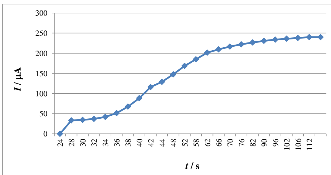
Slika 2. Ovisnost jakosti struje o vremenu difuzije za reakciju oksidacije apsorbiranih H-atoma u anodnom prostoru ( \text{H}^0 - e^- \rightarrow \text{H}^+ )
