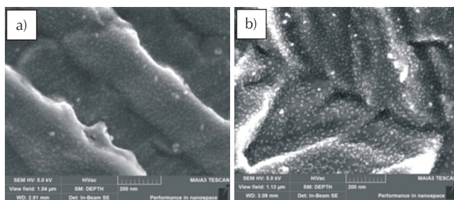
Slika 8 – SEM mikrografije legure s prisjetljivošću oblika Cu-12,8Al-4,1Ni u lijevanom (a) i kaljenom stanju 850 °C/60/ H 2 O (b), kod povećanja 260000× (a) i 240000× (b) 46
