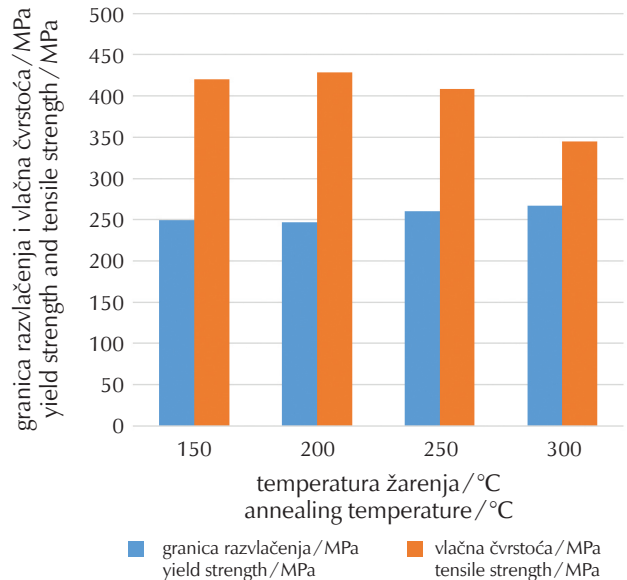
Slika 5 – Utjecaj temperature žarenja na granicu razvlačenja i vlačnu čvrstoću legure Cu-12,8Al-4,1Ni nakon austenitizacije i gašenja na 850 °C/60'/H 2 O 46
