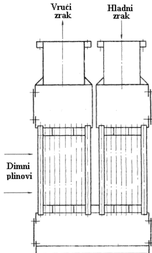
Slika 8. Izmjenjivač toplina od ravnih cijevi [15]
