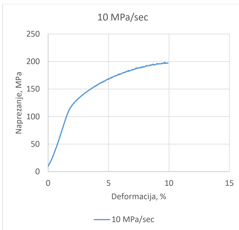
Slika 36. Dijagram naprezanje-deformacija s konstantnim porastom napreznja 10 MPa/s
