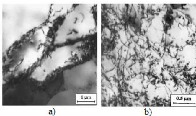
Slika 9. TEM prikaz gustoće dislokacija nakon istog stupnja deformacije kod (a) čistog aluminija, (b) aluminij-magnezij legure [29]
