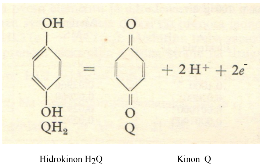
Slika 10: Strukturna formula kinona i hidrokinona [31]
