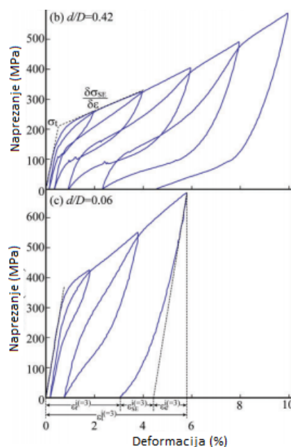
Slika 11. Krivulje naprezanje - deformacija dobivene od uzorka žice s različitim d/D [14]
