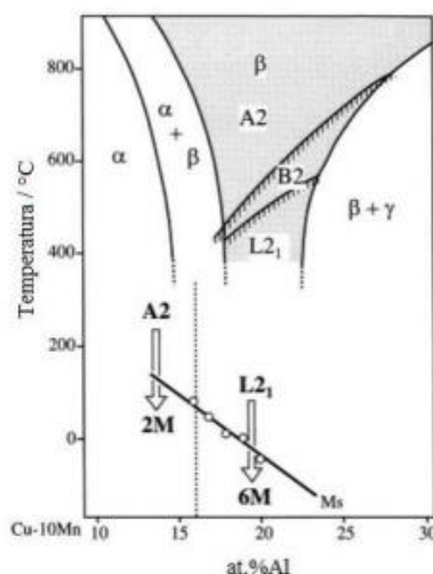
Slika 12. Vertikalni presjek faznog dijagrama CuAlMn legure pri 10 at.% Mn [39]
