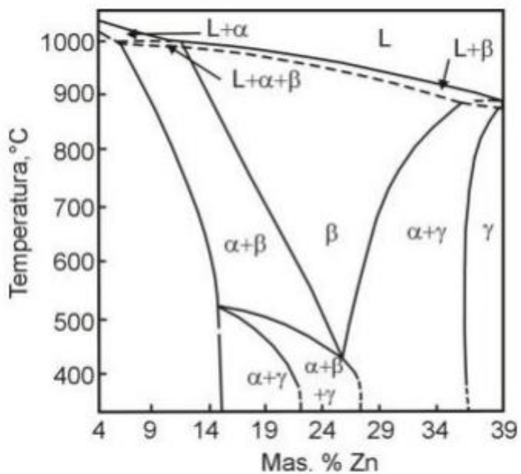
Slika 5. Fazni dijagram za Cu-Al-Zn leguru [14]
