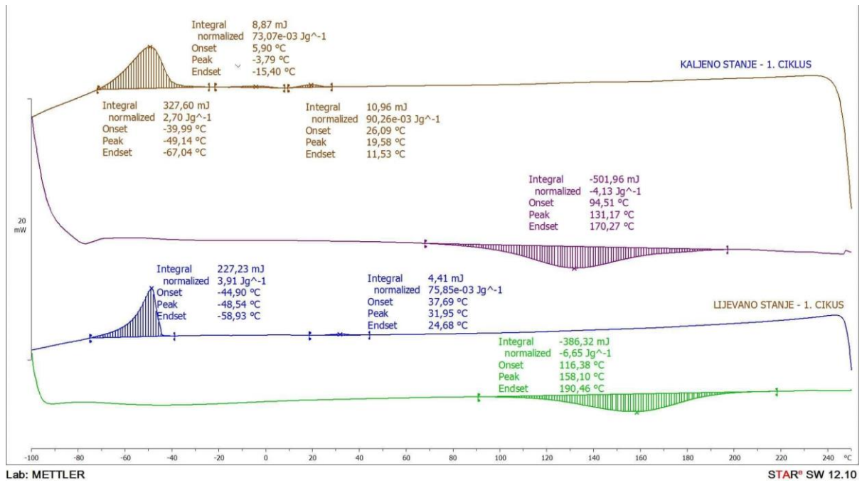
Slika 22. DSC termogram za Cu-9Al-10Mn-3Ag leguru nakon 1. ciklusa zagrijavanja/hlađenja u lijevanom i kaljenom stanju
