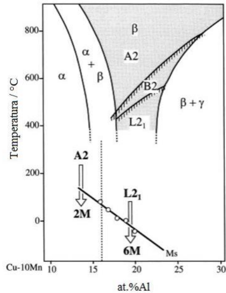
Slika 6. Vertikalni presjek Cu-Al-Mn legura pri 10 at.% Mn [16]
