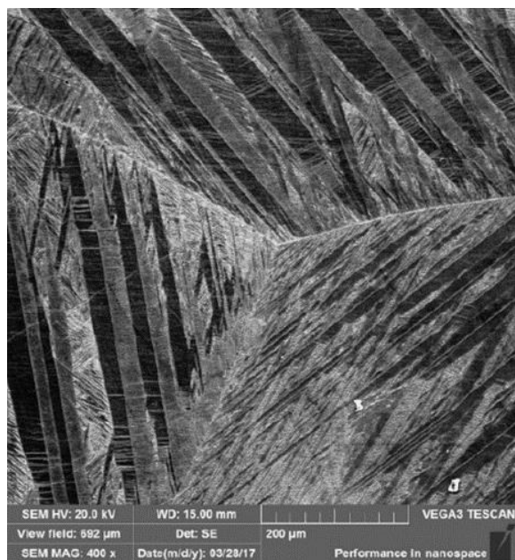
Slika 39. Mikrofotografija Cu10Al18Mn4Ag legure nakon betatizacije i kaljenja u vodi
