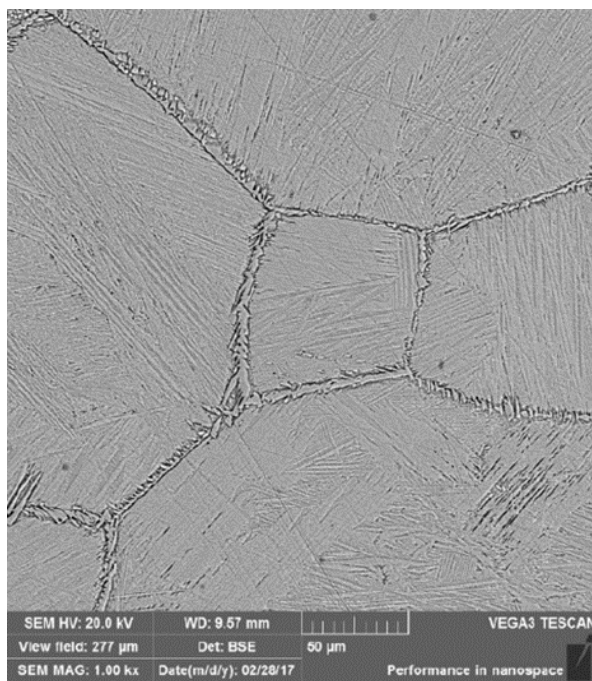
Slika 38. Mikrofotografija Cu10Al18Mn4Ag legure u lijevanom stanju
