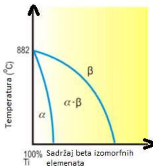
Slika 8. Utjecaj beta-izomorfnih elemenata na titan [18]
