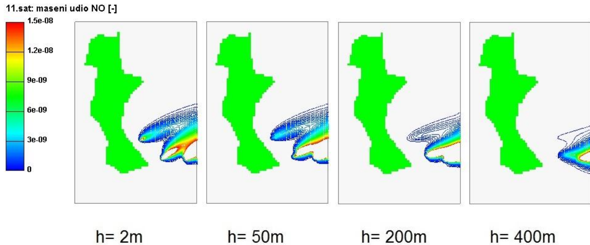
Slika 61. Prikaz dimnih perjanica u 11. satu za vrijednosti koncentracija NO
