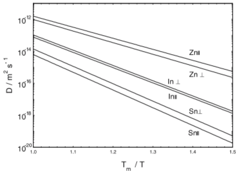
Slika 35. Dijagram samodifuzije u monokristalima Zn, In i Sn paralelno i okomito na osi ravnine [34]
