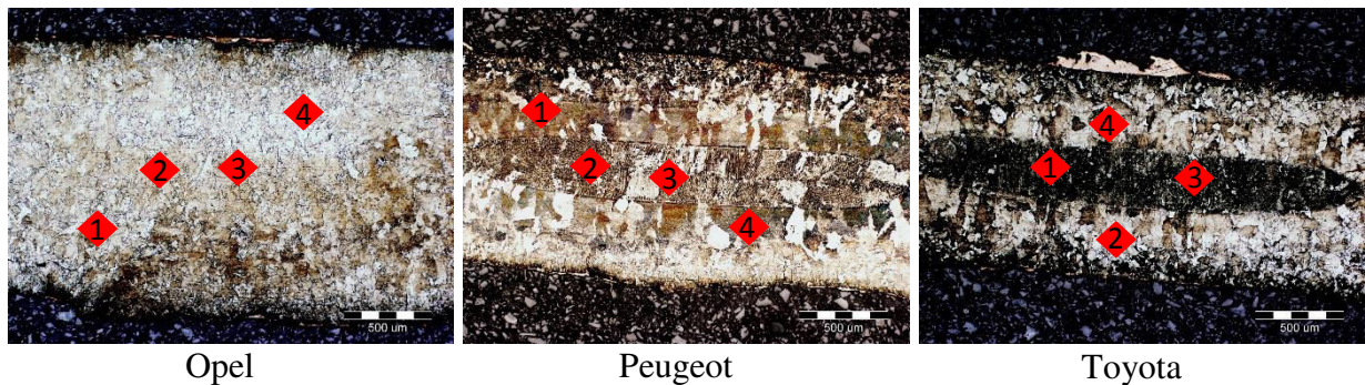
Slika 34. Mjesto mjerenja makro-tvrdoće na sva tri zavar
