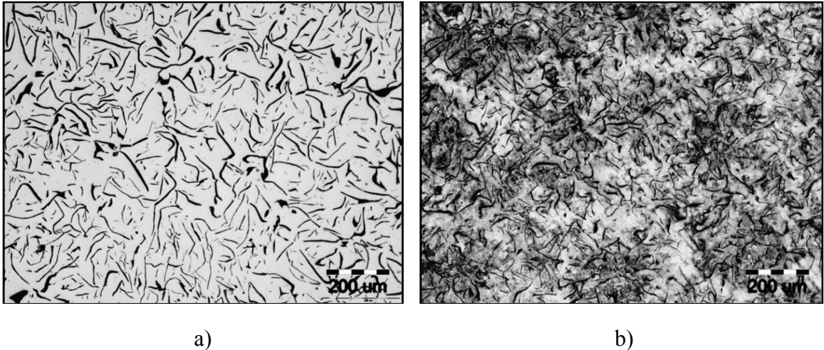
Slika 2.1. Mikrostruktura sivog lijeva: a) nenagrizenno stanje, b) nagrizenno stanje (sredstvo za nagrivanje – nital) [1]
