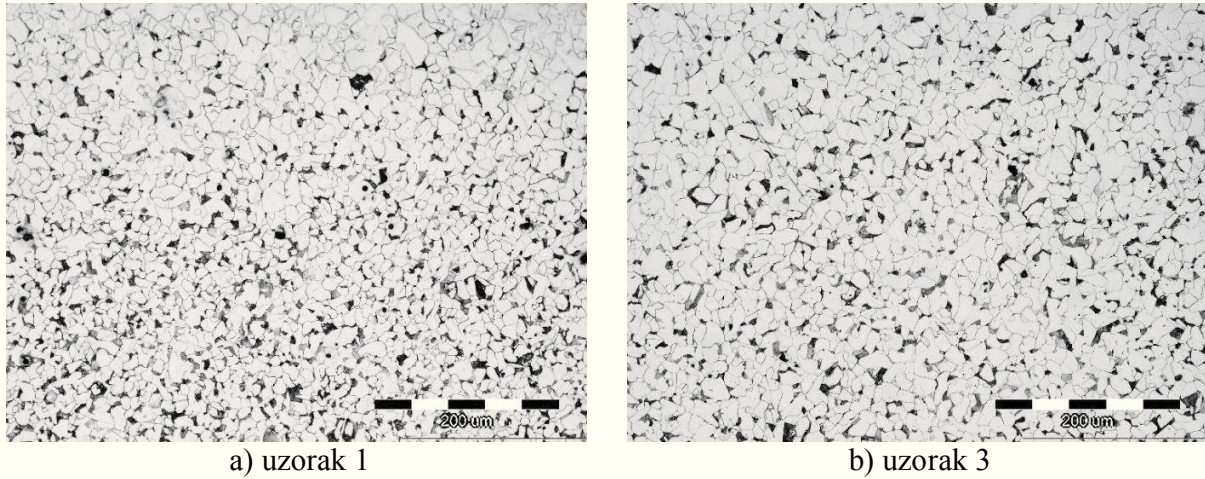
Slika 30. Metalografski snimci prijelaznog područja u uzorcima 1 i 3 pri povećanju 200x
