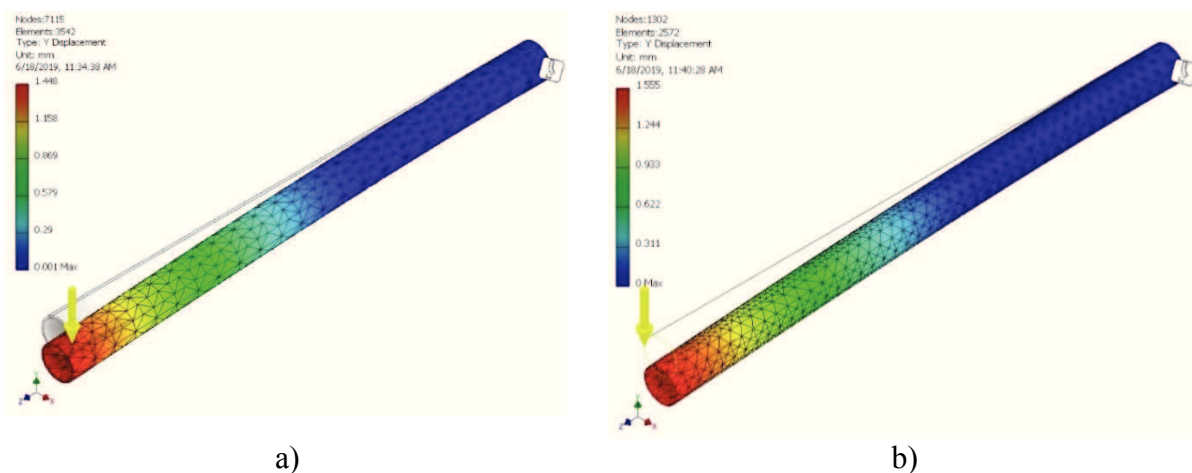
Slika 22. Rezultati progiba uz diskretizaciju: a) 3D tetraedarskim elementima, b) Shell elementima
