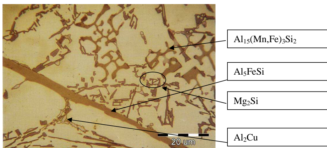
Slika 18. Mikrostruktura uzorka \text{AlSi9Cu3(Fe)} legure hlađenog brzinom 5^\circ\text{C/s} , pri povećanju 1100\times [9].
