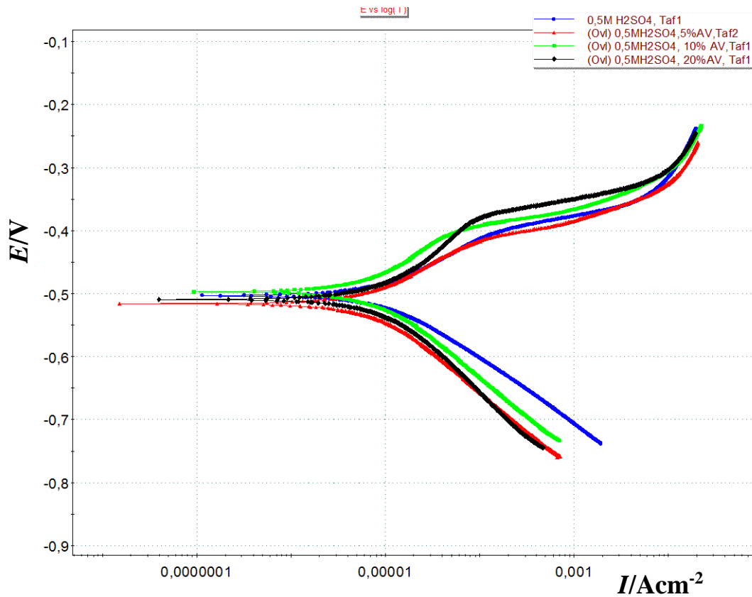
Slika 41. Polarizacijska krivulja ispitano konstrukcijskog čelika St.52.3 u različitim medijima pri temperaturi od 20 °C
