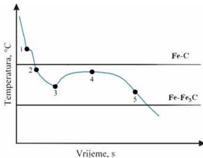
Slika 4. Shematski prikaz krivulje hlađenja podeutektičnog sivog lijeva [1]
