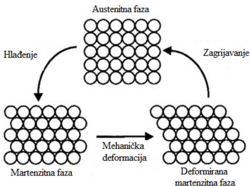
Slika 9. Prikaz martenzitne transformacije [12]
