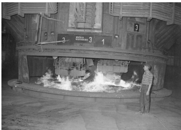
Gornji sloj peći za proizvodnju ferolegura, Tvornica karbida i ferolegura Dalmacija – Dugi Rat, druga polovica XX. st.
