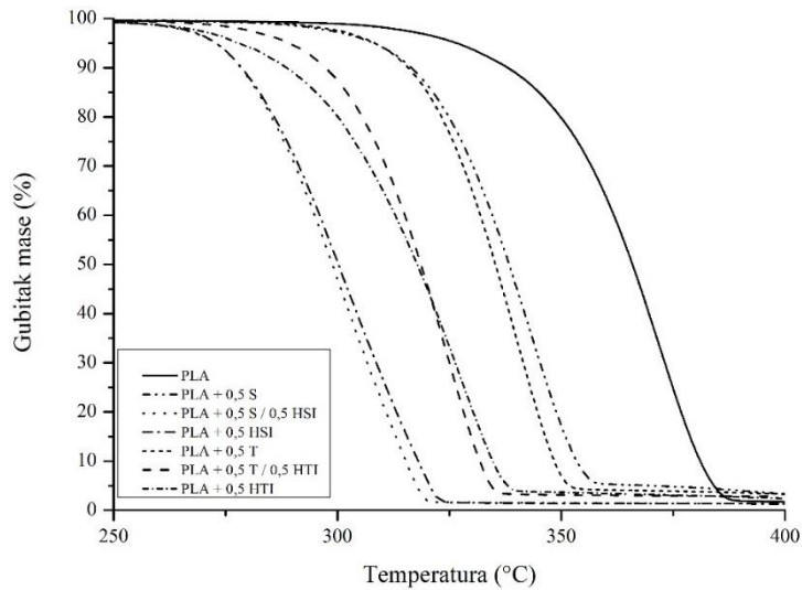
Slika 4. Termogravimetrijska krivulja PLA polimera i PLA kompozita.
