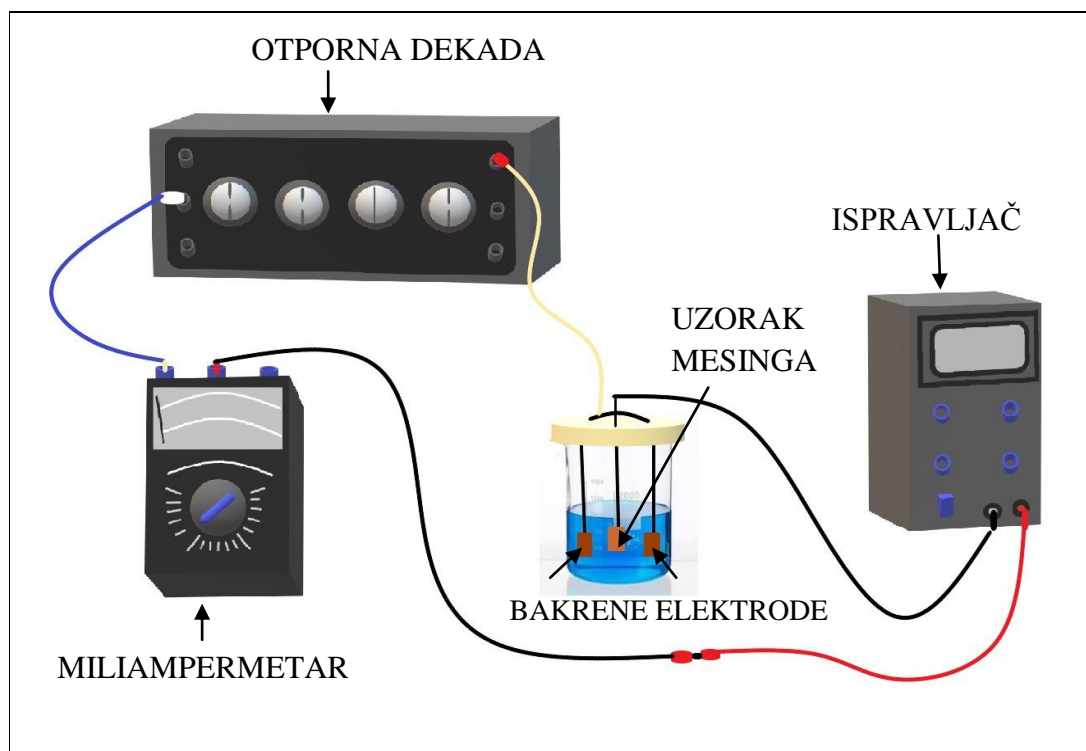
Slika 1. Skica aparature za nanošenje prevlake bakra metodom elektrodepozicije i za određivanje iskorištenja struje [*]
